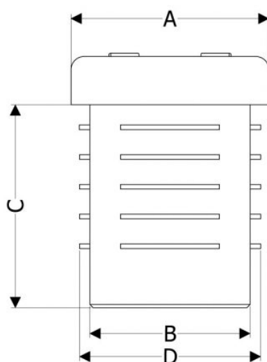
Wymiary wkładki z gwintem M8
